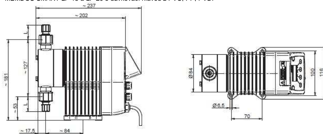
MEMDOS SMART LP 5 - LP 20 s dávkovací hlavou z nerezové oceli
