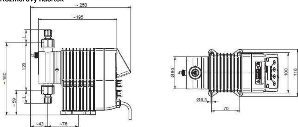
MEMDOS SMART LP 5 a LB 10 s dávkovací hlavou z PVC, PP, PVDF
