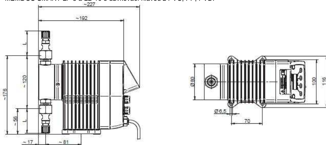
MEMDOS SMART LP 15 a LP 20 s dávkovací hlavou z PVC, PP, PVDF
